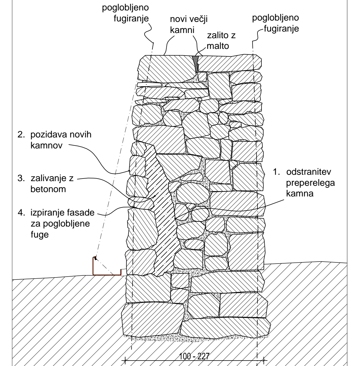
PREREZ ZIDU NA LOKACIJAH POTREBNIH OBNOVE M1:20
