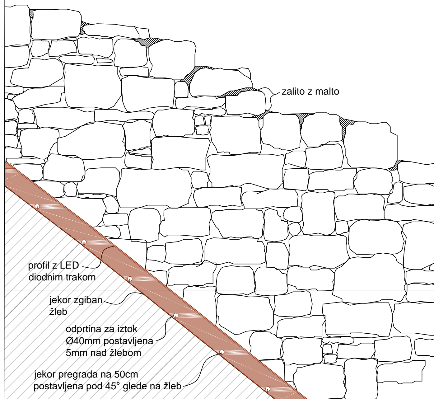
POGLED NA ZID M1:20
