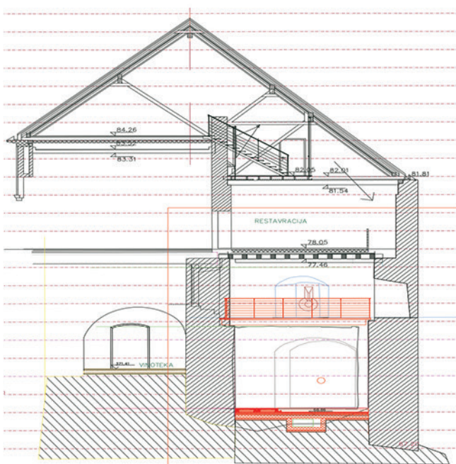
PREČNI PREREZ D3-D3
