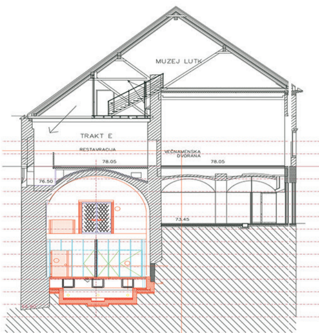
PREČNI PREREZ D2-D2
